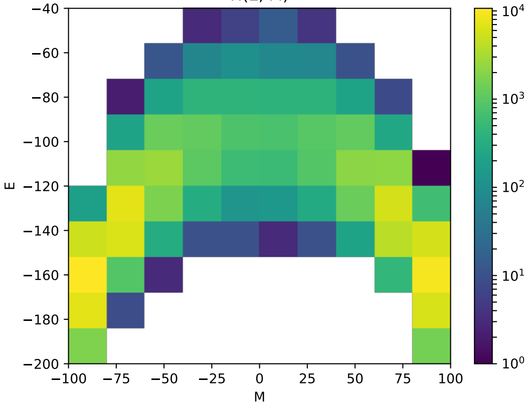
H(E, M)
